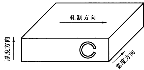
图 A.2 压延产品的 C 环取样图
