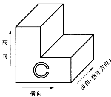
图 A.1 挤压产品的 C 环取样图
